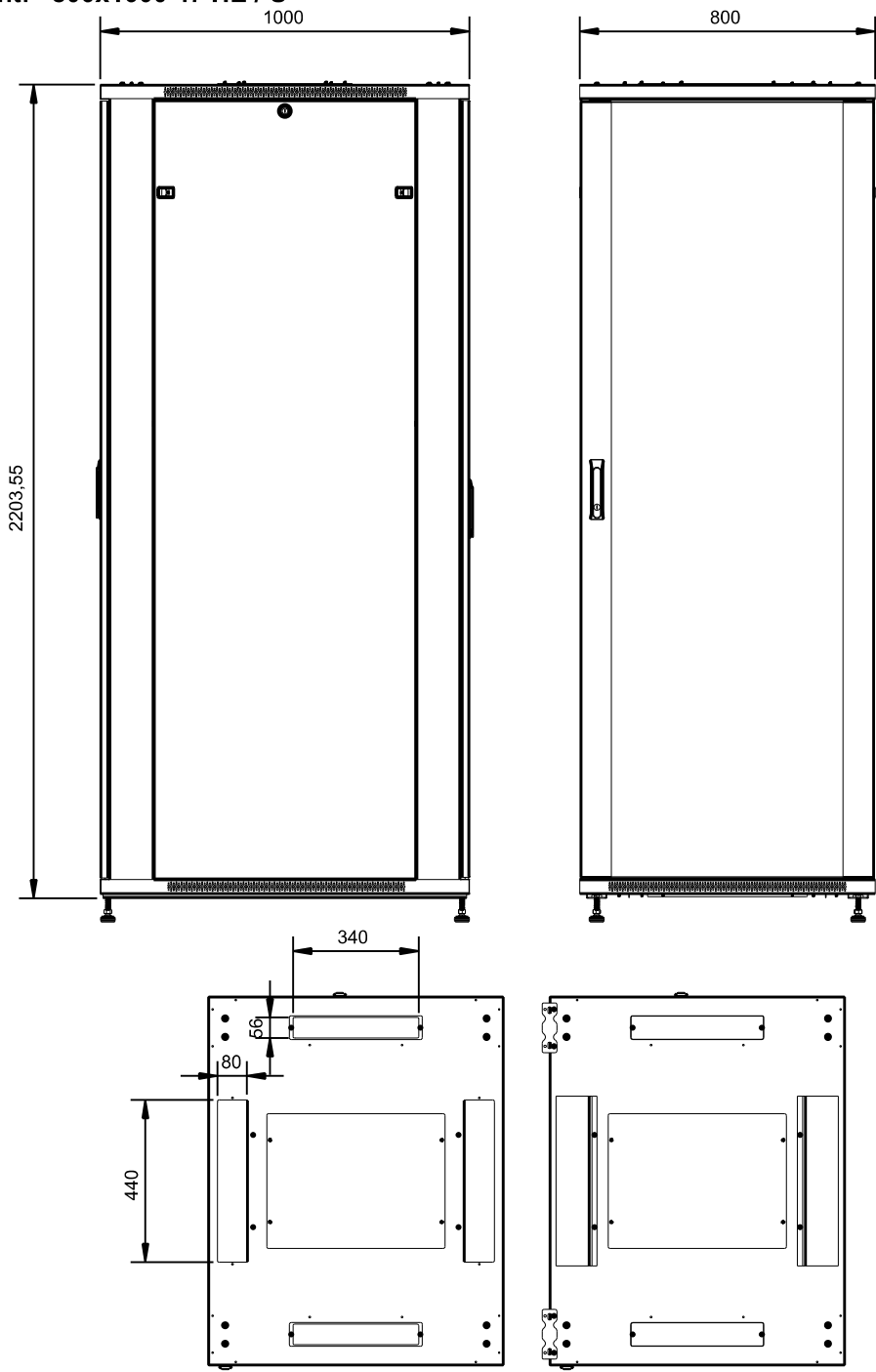
Ansicht oben / Top view ohne Verbindungselement / w/o connecting element Kabeleingänge ohne Abdeckung / Cable entries without covers Ansicht oben / Top view mit Verbindungselement / with connection element mit Bürsten / with brush strips
