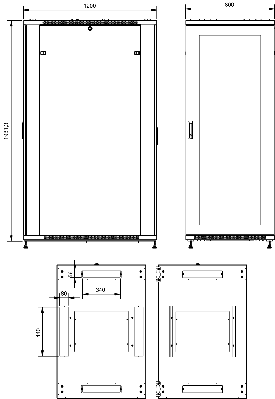
Ansicht oben / Top view ohne Verbindungselement / w/o connecting element Kabeleingänge ohne Abdeckung / Cable entries without covers Ansicht oben / Top view mit Verbindungselement / with connection element mit Bürsten / with brush strips
