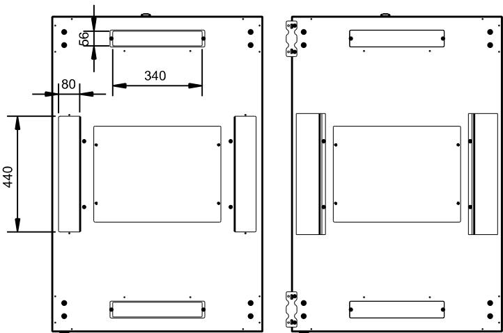
Ansicht oben / Top view ohne Verbindungselement / w/o connecting element Kabeleingänge ohne Abdeckung / Cable entries without covers Ansicht oben / Top view mit Verbindungselement / with connection element mit Bürsten / with brush strips
