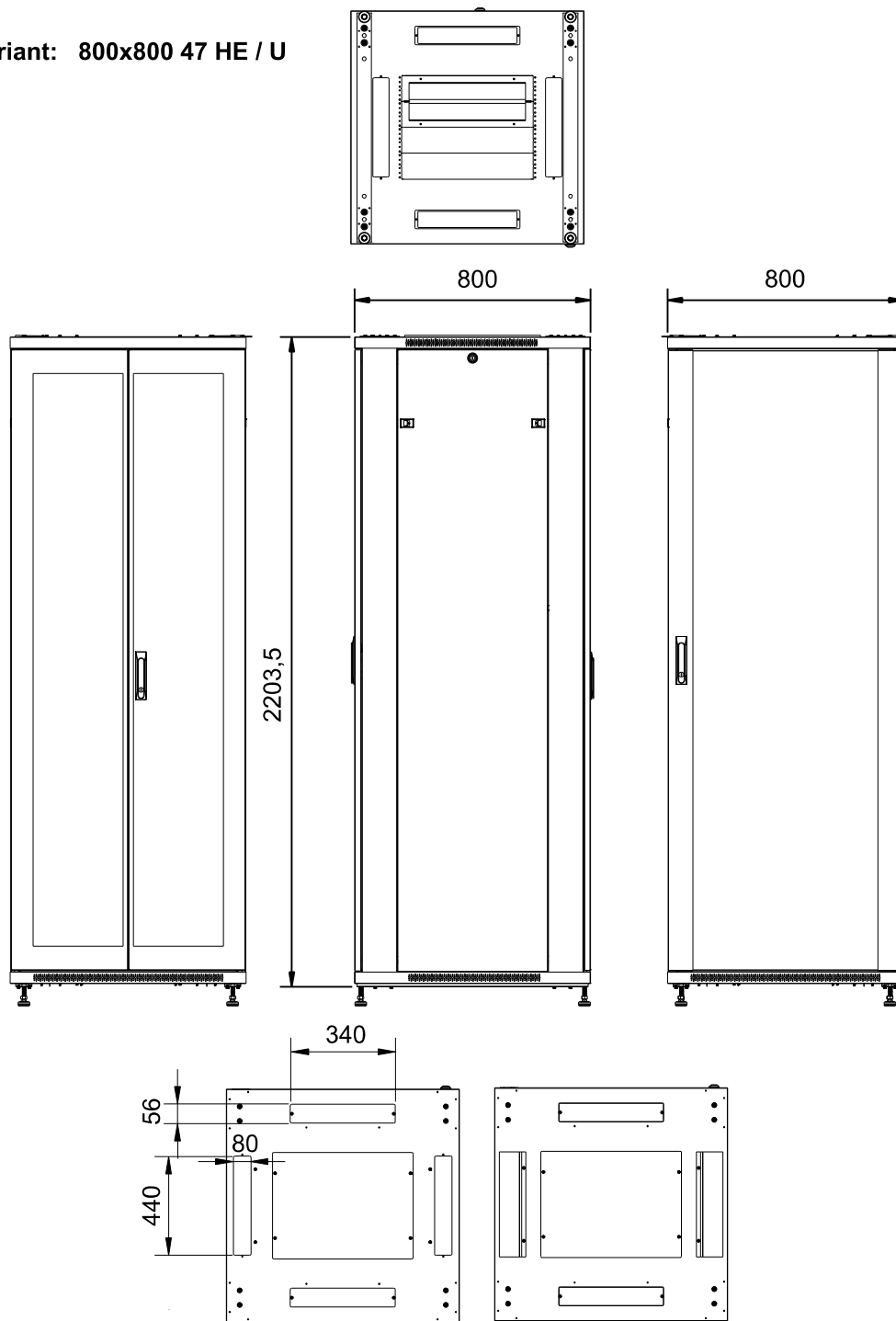
Ansicht oben / Top view Kabeleingänge ohne Abdeckung / Cable entries without covers Ansicht oben / Top View mit Bürsten / with brush strips
